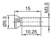
1430 Torx T-8
