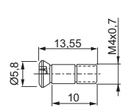
1635 Torx T-10
