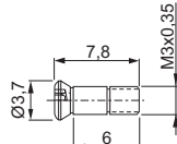
1435 Torx T-15
