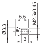
1425 Torx T-7
