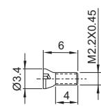
1639 Torx T-25
