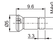
1445 Torx T-15
