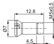
1622 Torx T-7
