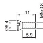
1629 Torx T-20
