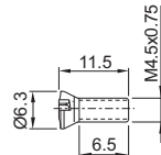
1353 Torx T-8
