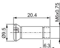
1630 Torx T-9
