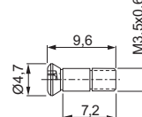
1440 Torx T-15
