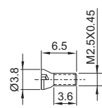
1640 Torx T-15
