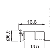
1649 Torx T-30
