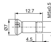
1625 Torx T-8
